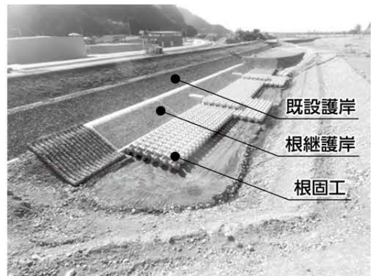
姫川（西中地先）における急流河川対策
