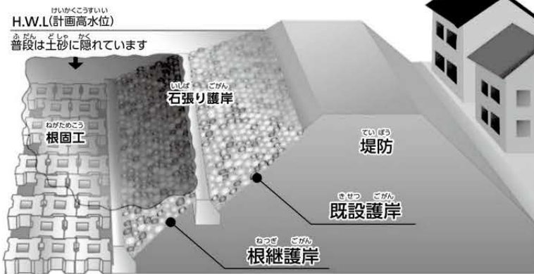
姫川（西中地先）における急流河川対策
