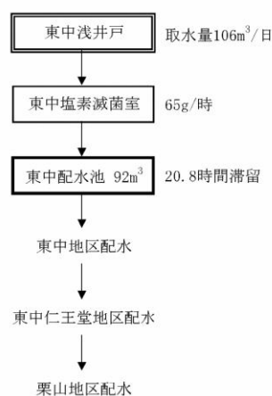
別図 1-5 姫川簡易水道事業の施設フロー
