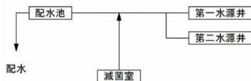
別図 1-13 市振簡易水道事業の施設フロー
