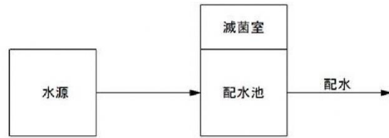
別図 1-14 上路簡易水道事業の施設フロー
