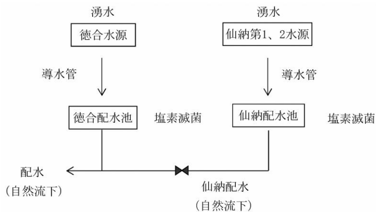
別図 1-11 徳合仙納簡易水道事業の施設フロー
